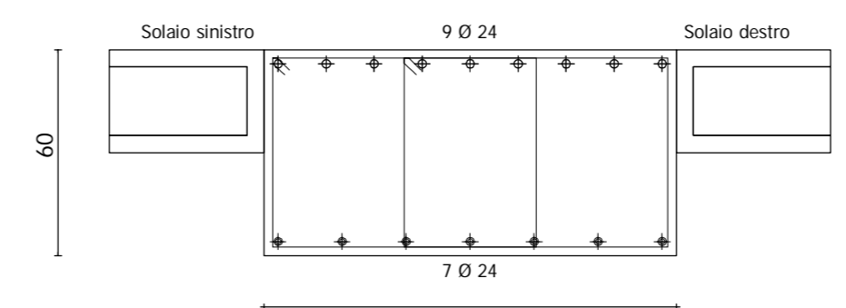
Sezione B - B - 1:20
