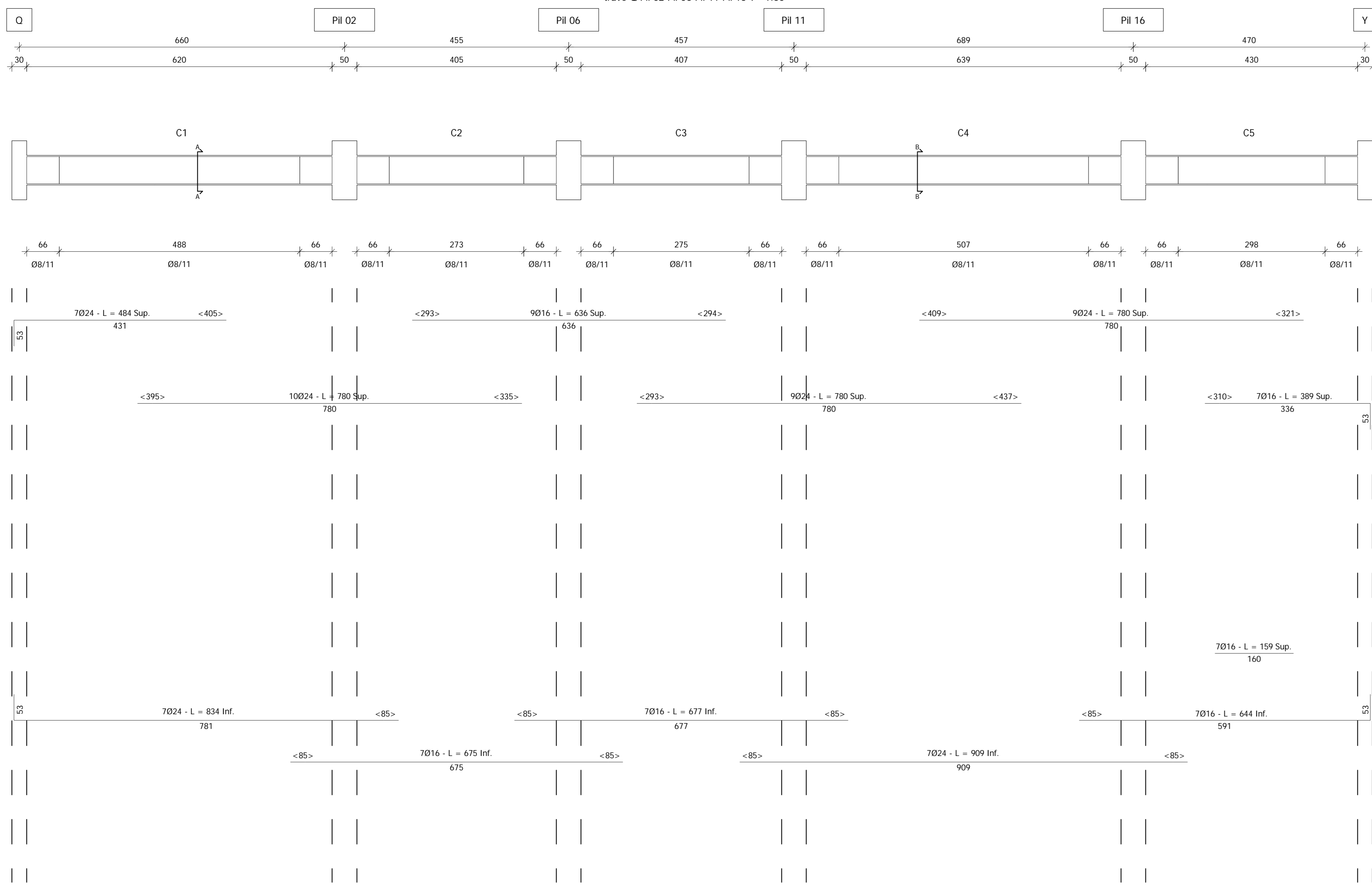
- trave Q Pil 02 Pil 06 Pil 11 Pil 16 Y - 1:50
