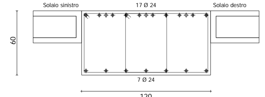
Sezione A - A - 1:20
